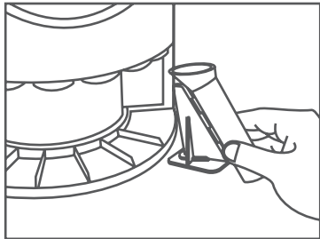
Figura 2 - Instalación del tubo de monedas
