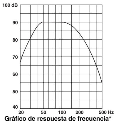
Gráfico de respuesta de frecuencia*
