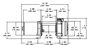
Figure 2. Winch dimensions: 10.3" L. x 4.0" D. x 4.56" H. 26cm L. x 10cm D. x 11cm H.
