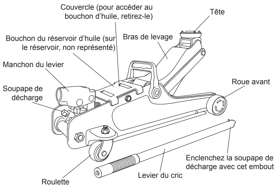
Figure 1 - Nomenclature typique du cric rouleur
