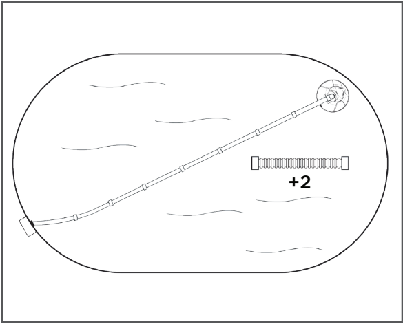
3B Determine el largo de la manguera
