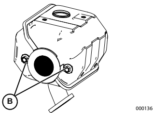
Figure 4-10. Fixations du pare-étincelles
