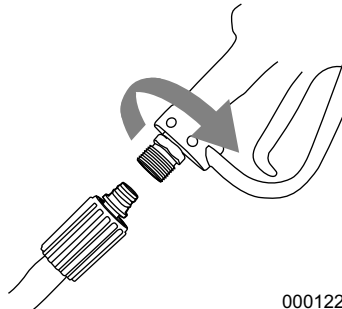
Figura 2-12. Conexión de la manguera de alta presión a la pistola de pulverización
