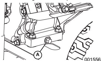
Figura 4-7. Tapón de vaciado de aceite
