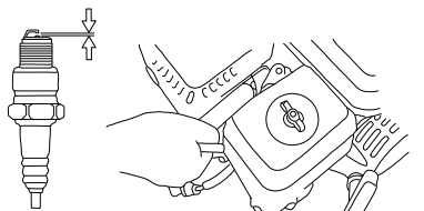
Figura 4-8. Bujía
