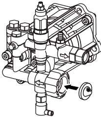
Figura 2-8. Inspección del tamiz de entrada
