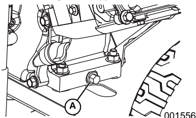
Figure 4-7. Bouchon de vidange de l'huile
