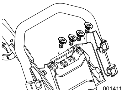
Figura 2-3. Inserción de las boquillas
