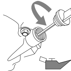
Figura 4-5. Llenado de aceite de motor
