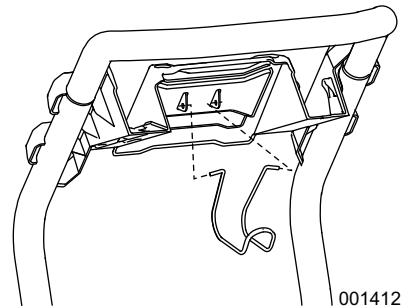
Figure 2-2. Installation du crochet du tuyau
