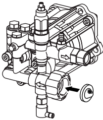
Figure 2-8. Inspection du tamis de la prise d'eau
