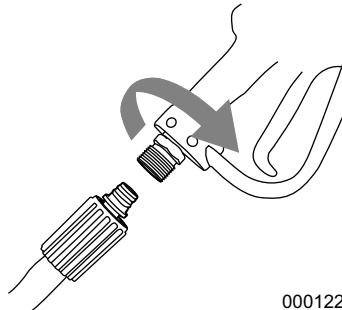
Figure 2-12. Raccord du tuyau à haute pression au pistolet de pulvérisation
