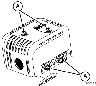
Figura 4-9. Fijaciones del protector de calor
