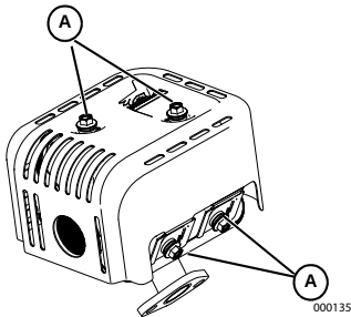
Figure 4-9. Fixations de l'écran thermique
