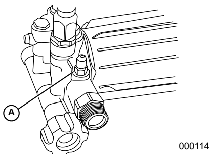
Figure 2-4. Fixation du tube de siphonnement
