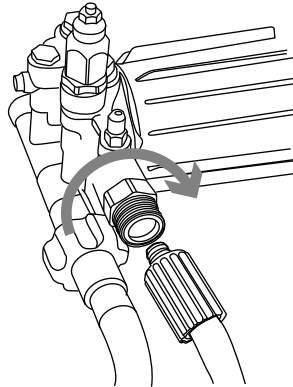
Figura 2-11. Conexión de la manguera de alta presión a la bomba
