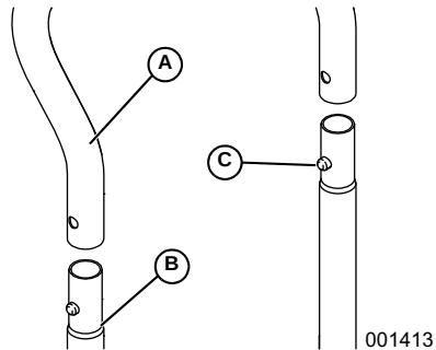
Figure 2-1. Insertion de la poignée
