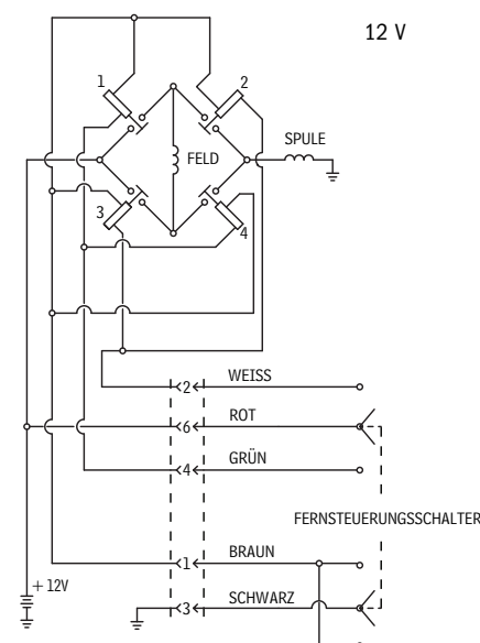
ELEKTRISCHES SCHALTBIKD
