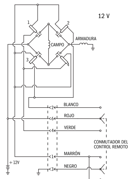
ESQUEMA DEL CIRCUITO ELÉCTRICO
