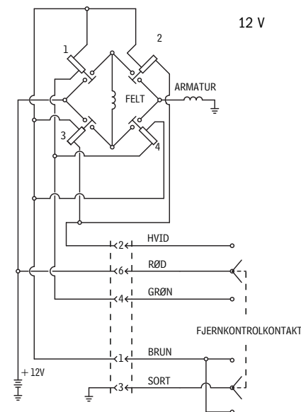
ELEKTRISK KREDSLØBSDIAGRAM
