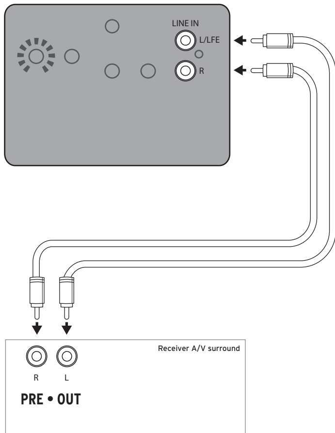
FIGURA 2 CONEXÃO DO SUBWOOFER R-10SW, R-12SW
