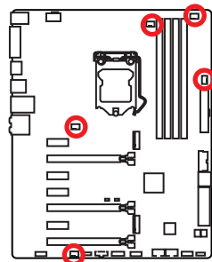
PWM Mode fan connector
