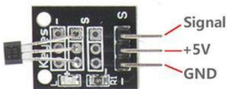
Linear Hall
