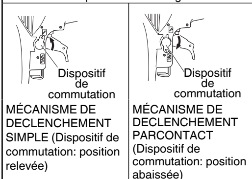
Dispositif de commutation d'opération de clouage
