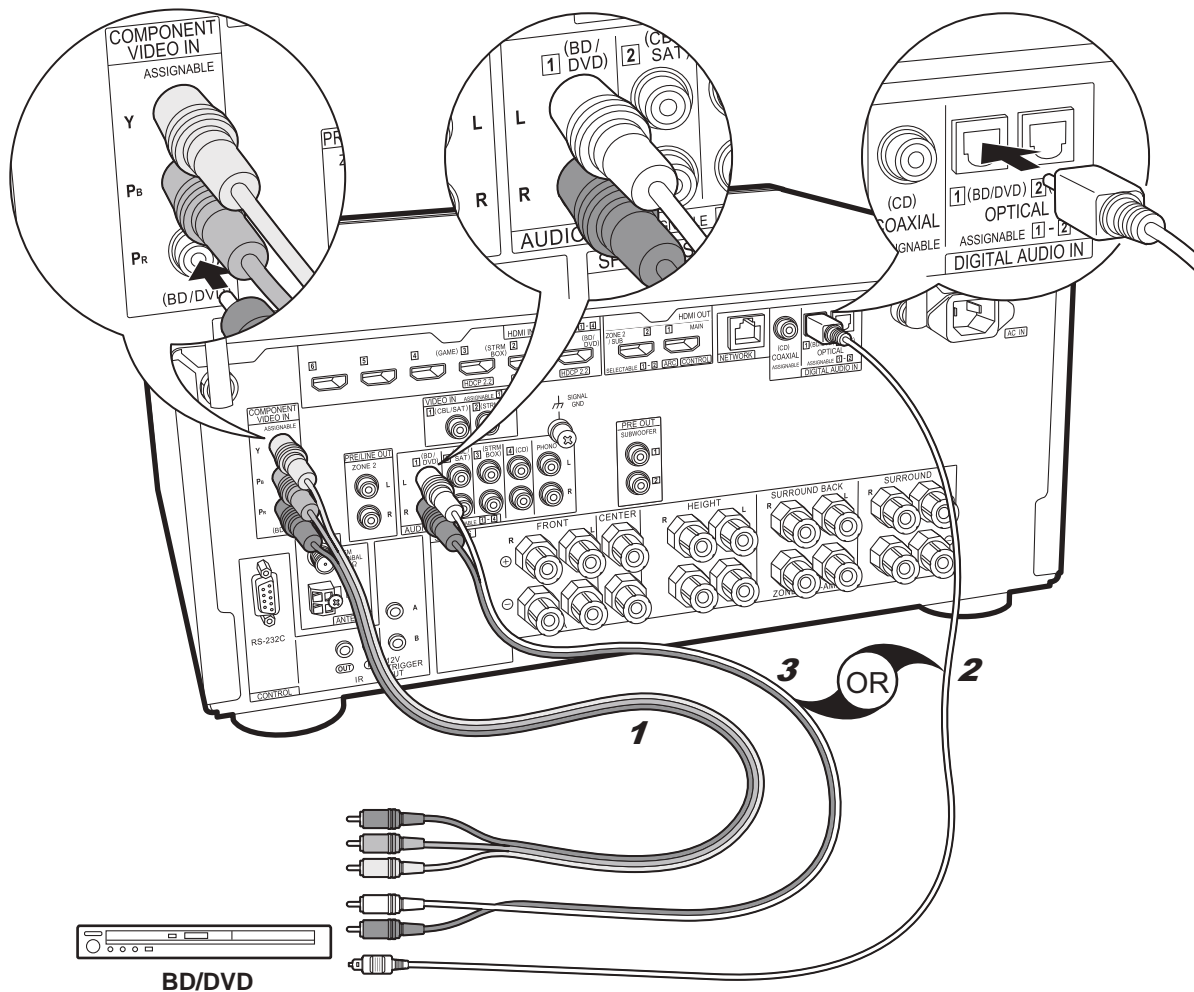
1 Câble vidéo composante, 2 Câble optique, 3 Câble audio analogique
