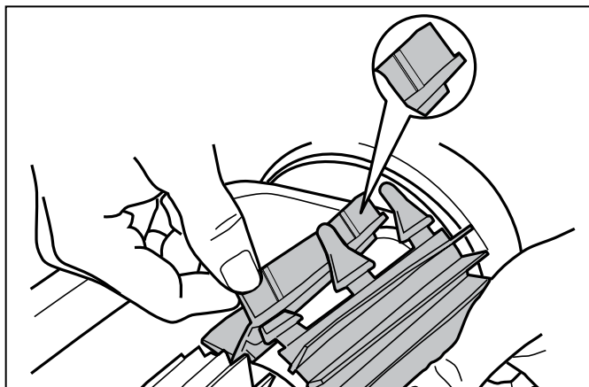
Figure 29. Témoins d'usure
