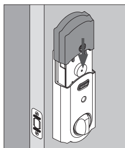
3. Vuelva a colocar la bandeja de las baterías con las baterías mirando hacia la puerta. Coloque el conector de las baterías en la bandeja y vuelva a colocar la cubierta.
