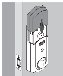
3. Remettez le support de piles en place, les piles orientées vers la porte. Rebranchez le connecteur au support de piles et remplacez le couvercle.
