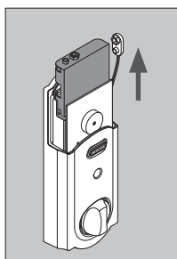
2. Destrahe el conector de las baterías, retire la bandeja de las baterías y cámbielas.
