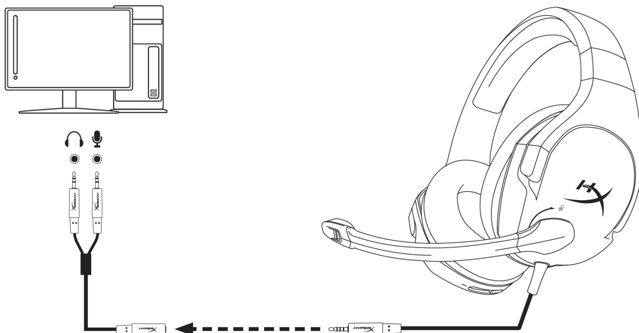
Uso con alargador para PC
