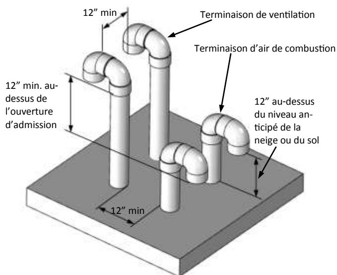
Terminaison verticale de plusieurs chauffe-eau
