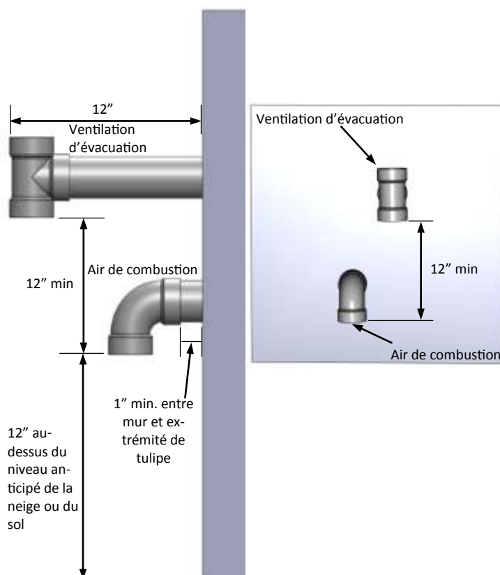
Terminaison avec té pour tuyauterie de ventilation et d'air de combustion sur mur de côté
