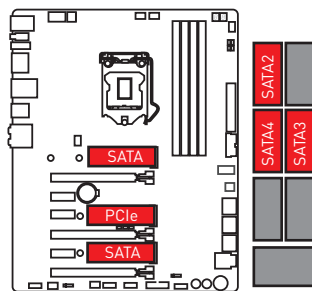
2xM.2 SATA SSDs + 1xM.2 PCIe SSD+ 3xSATA HDDs
