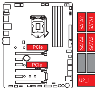
2xM.2 PCIe SSDs + 1x U.2 SSD + 4xSATA HDDs
